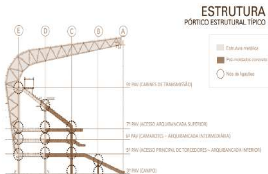
Figura 01 – Pórtico estrutural típico da Arena MRV
